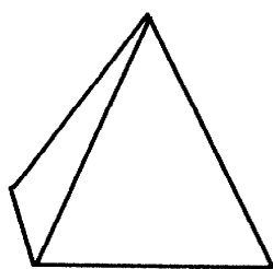
tetraedre
