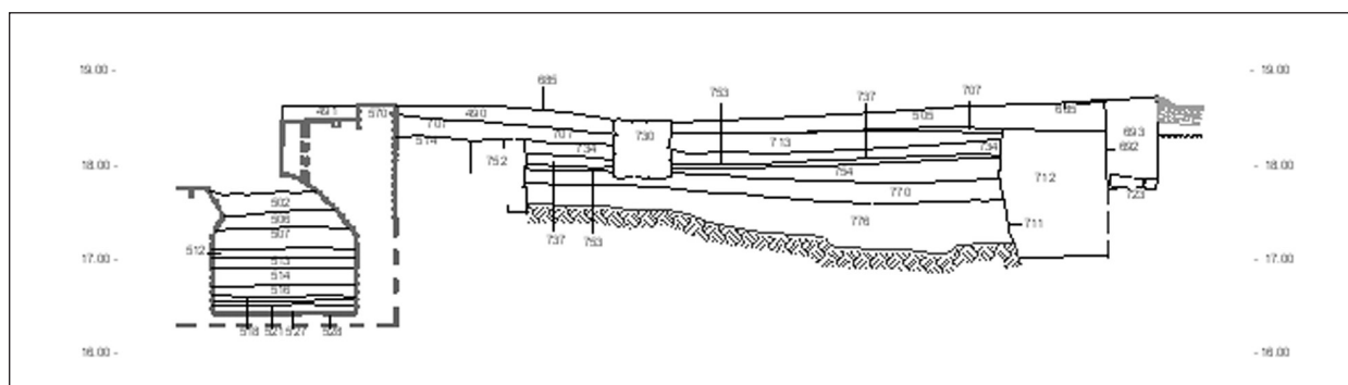
FIGURA 23. Secció estratigràfica del jaciment.
