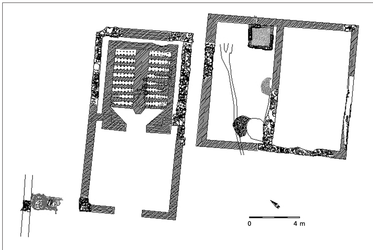
FIGURA 32. Restitució hipotètica de la planta de les restes localitzades de la figlina .
