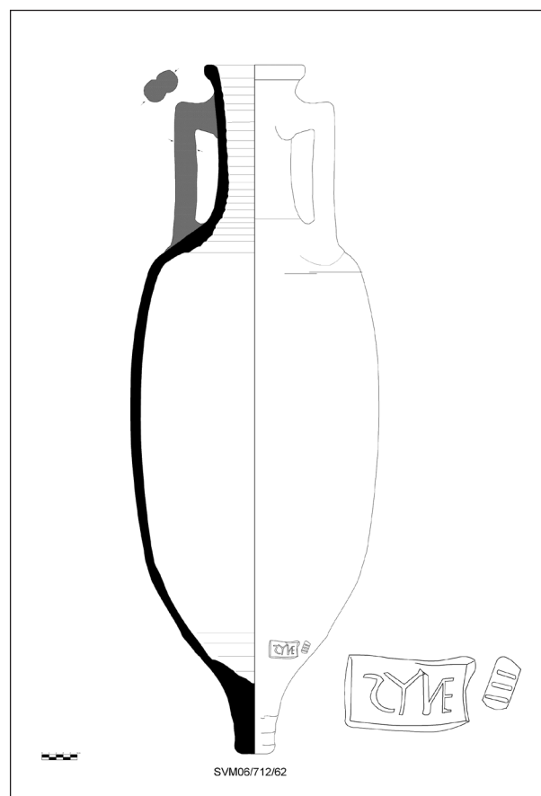
FIGURA 27. Àmfora Dressel 2-4 localitzada durant l'excavació.
